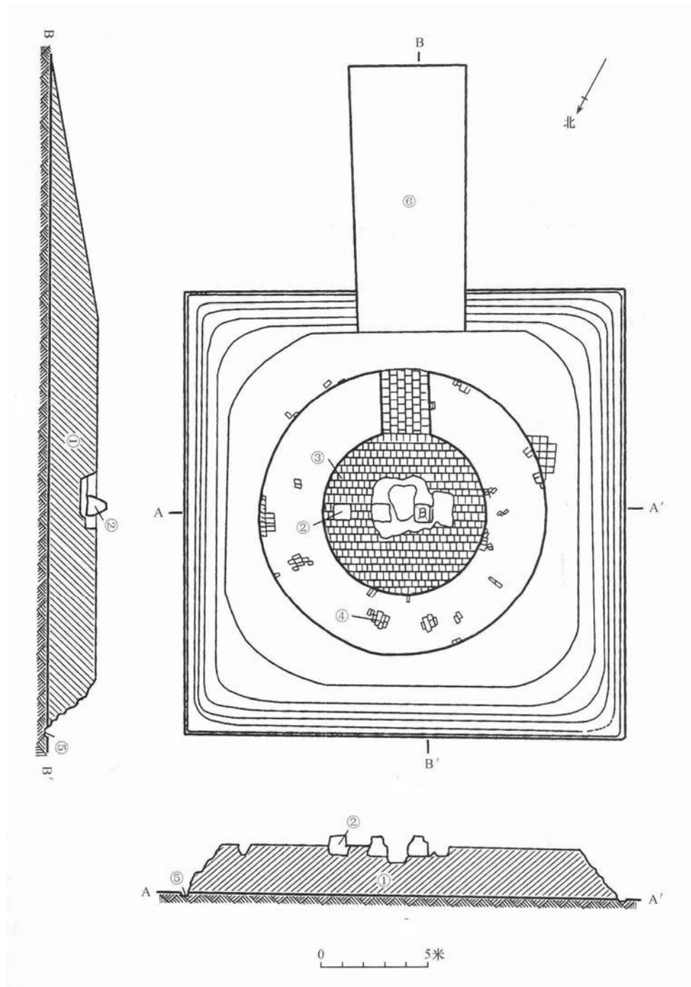
图四 西夏陵三号陵西碑亭平，剖面图
