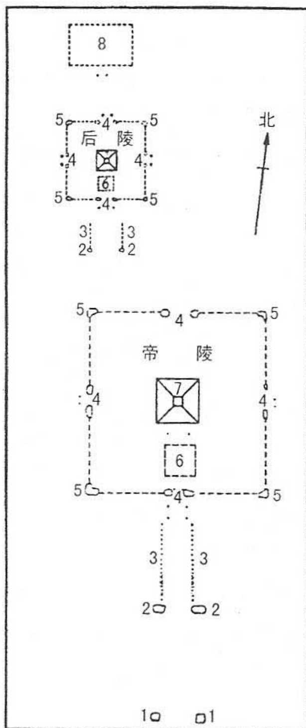
图二 北宋皇陵永定陵平面图
