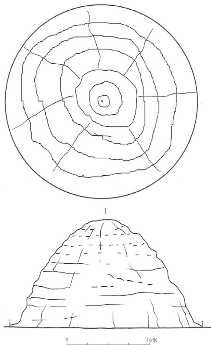
图六 西夏三号陵陵塔平，立面示意图
