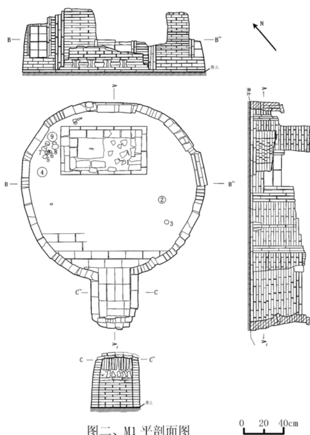
图二、M1 平剖面图
