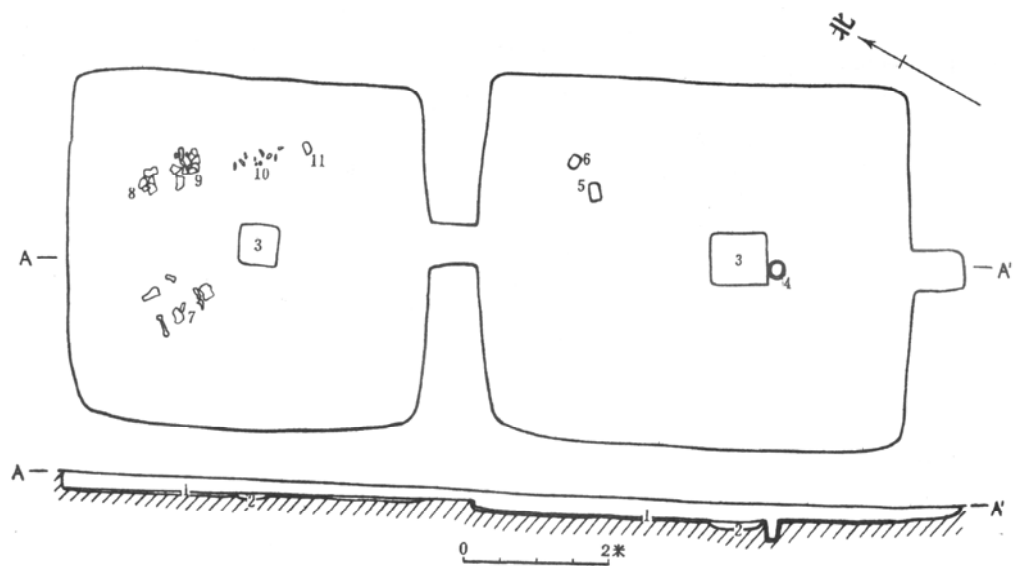
图一〇 南台子遗址 F24 平剖面图
