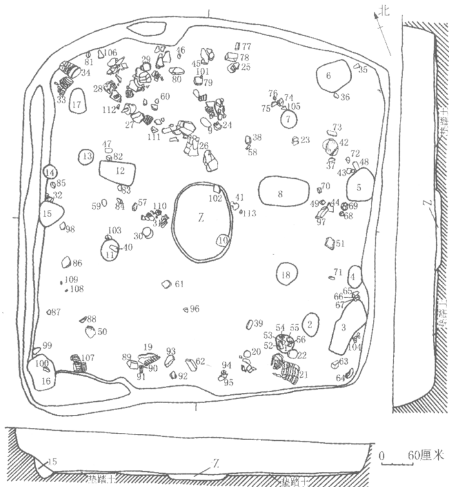
图一三 查海遗址 F54 平剖面图
