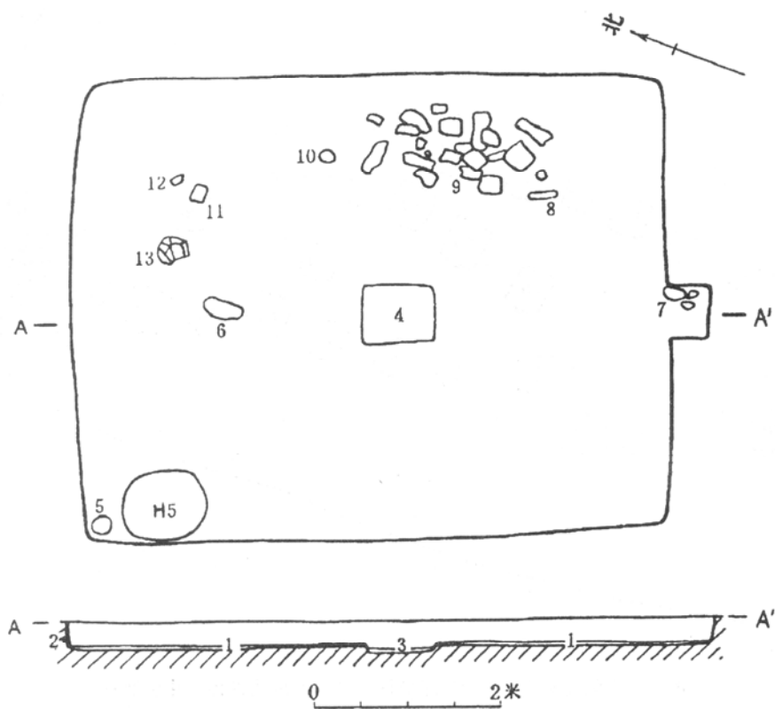
图六 南台子遗址 F2 平剖面图
