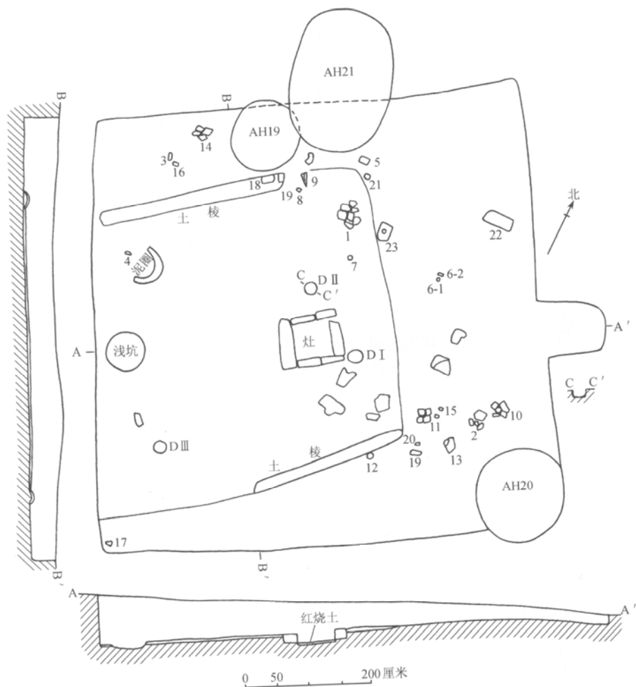
图七 白音长汗遗址 AF25 平剖面图
