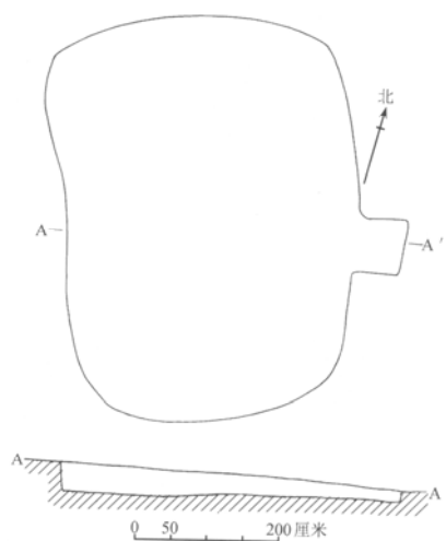
图八 白音长汗遗址 AF15 平剖面图
