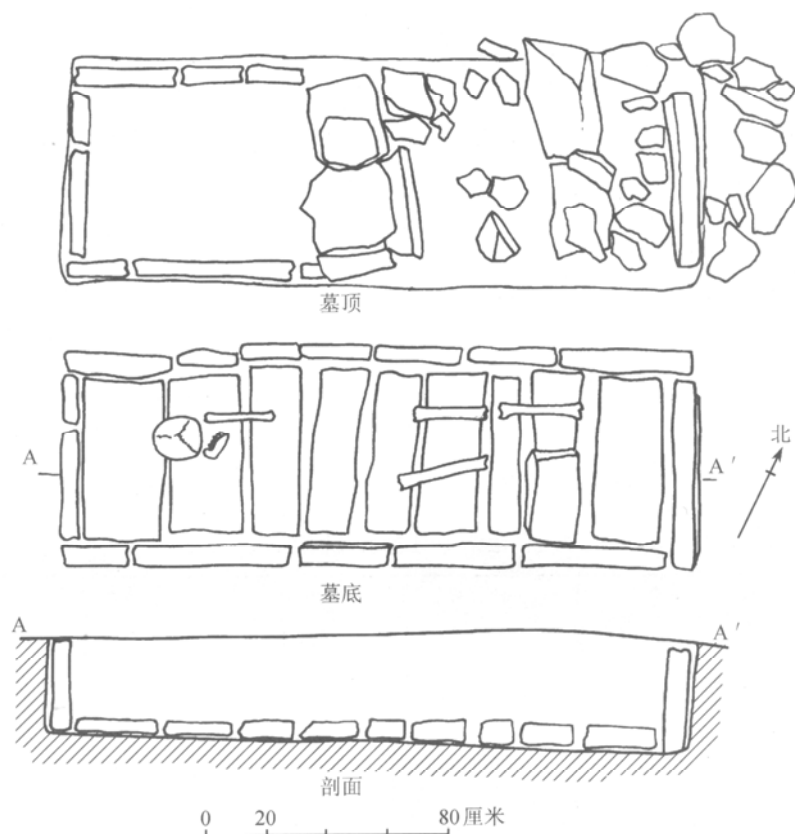
图一七 白音长汗遗址 M5 平剖面图
