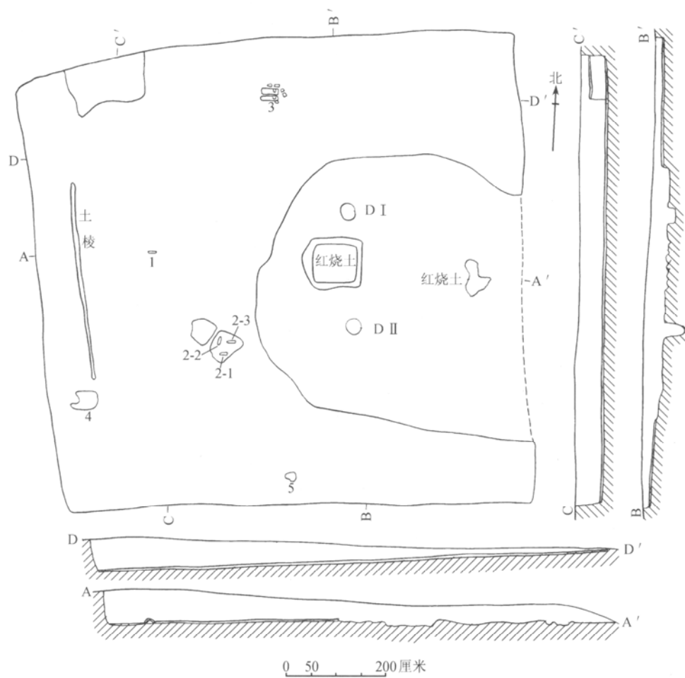
图一四 白音长汗遗址 AF68 平剖面图
