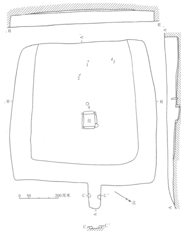
图一二 白音长汗遗址 AF19 平剖面图
