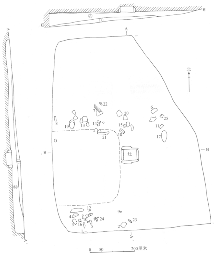
图九 白音长汗遗址 BF74 平剖面图
